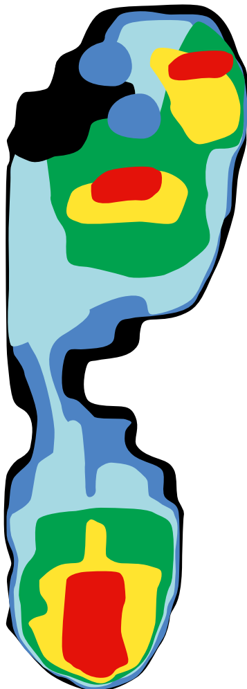
Druckverteilung im Schuh (rot = hohe Druckbelastung) // Pressure distribution in the shoe (red = high pressure load)
